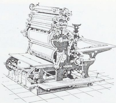
U NE ROTATIVE, LA ROTO-CALCO, FABRIQUÉE CHEZ VOIRIN EN 1910, AVANT QUE MARINONI N'ABSORBE CETTE ENTREPRISE.
